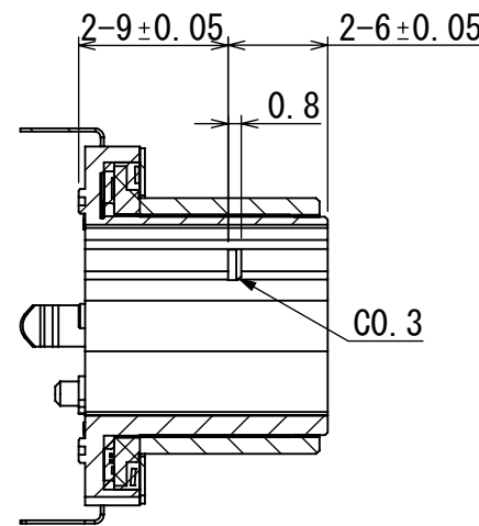
断面図 Y-Y SECTION Y-Y
