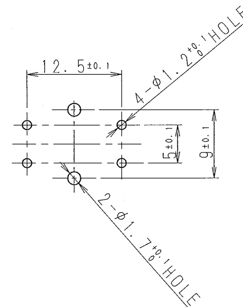
プリント基盤取付穴寸法 (スイッチ取付面側より見る) P.C BOARD MOUNTING HOLE DIMENSIONS (WHEN VIEWED FROM SWITCH MOUNTING FACE)
