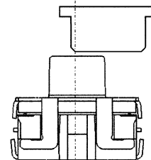
Fig 2: Set knob vs stem 図2: キートップとステムの関係
