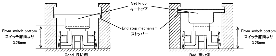
Fig. 3: End stop mechanism at module level (example) 図3: ストッパー位置の例
