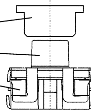
Fig 2: Set knob vs stem 図2: キートップとステムの関係
