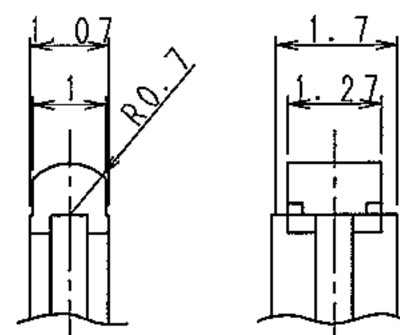
DETAIL A (10:1)
