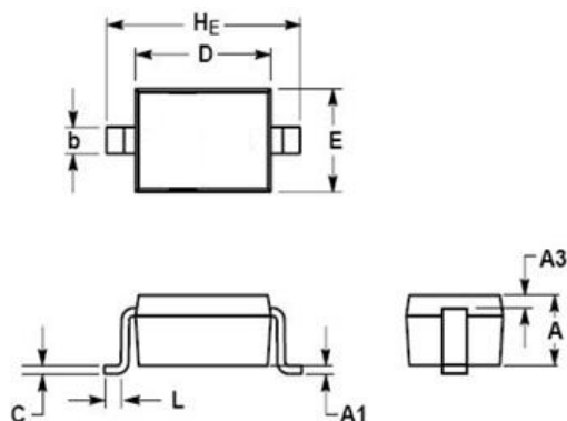
SOD323
