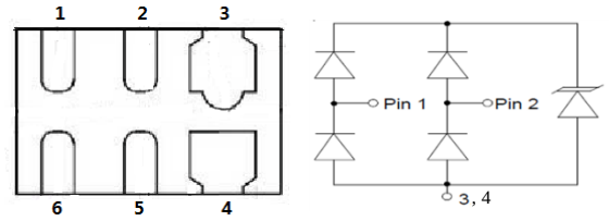
DFN1610-6L
