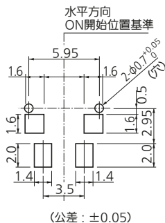
プリント基板取付穴参考図
