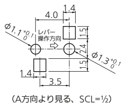
プリント基板取付穴参考図
