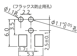
プリント基板取付穴参考図
