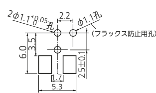
プリント基板取付穴参考図
