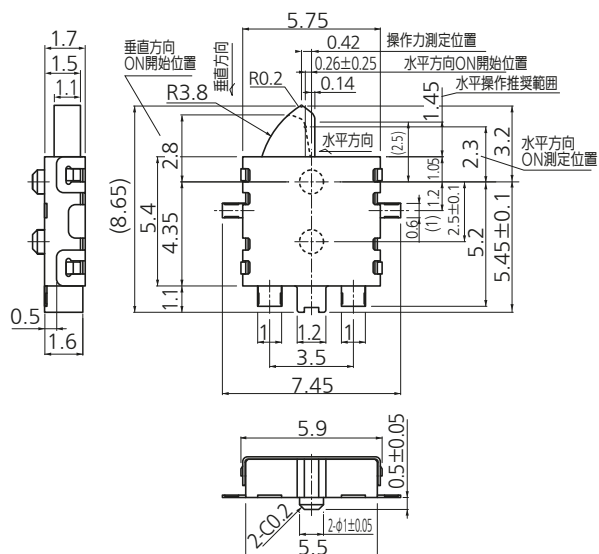
外形寸法図
