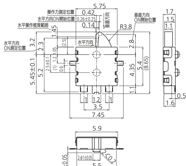
外形寸法図
