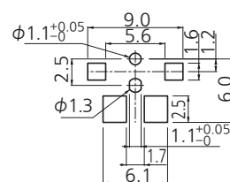
プリント基板取付穴参考図
