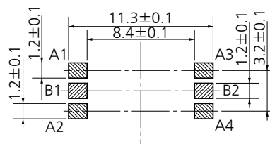
プリント基板パターン参考図
