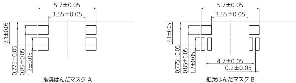
推奨はんだマスク
