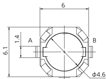
外形寸法図
