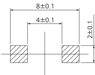
プリント基板パターン参考図
