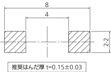
プリント基板パターン参考図
