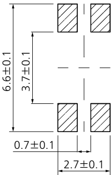
プリント基板パターン参考図
