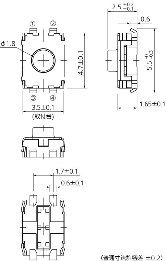
外形寸法図
