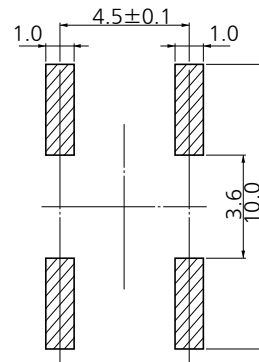
プリント基板取付穴参考図
