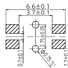
プリント基板パターン参考図
