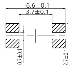
プリント基板パターン参考図
